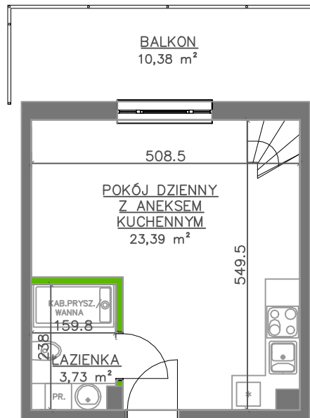
MIESZKANIE
